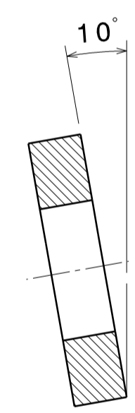
sez. C-C Scala: 5:1
